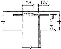
(e) 顶层中间节点柱筋90°弯折锚固
