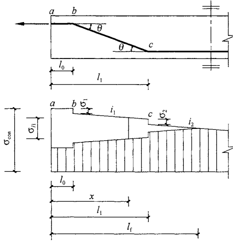
图 J.0.3-3 折线形预应力筋的预应力损失 \sigma_{n1}
